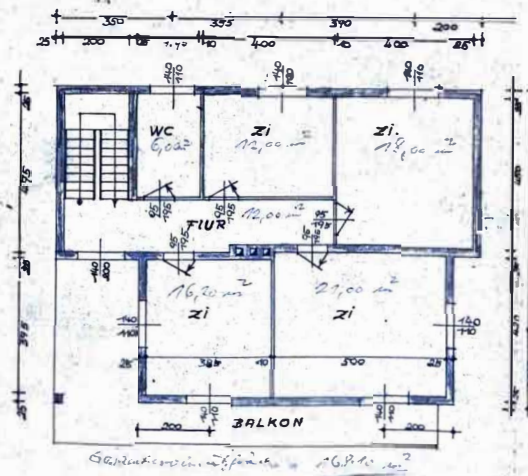
OBERGESCHOSS
