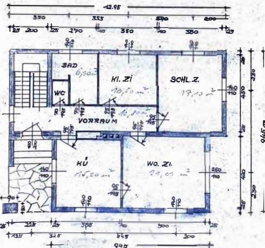
ERDGESCHOSS
