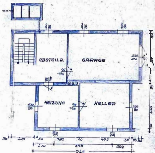
KELLERGESCHOSS
